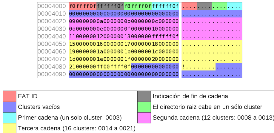
Figura 7.7: Ejemplo de entradas en la tabla de asignación de archivos en FAT32.
