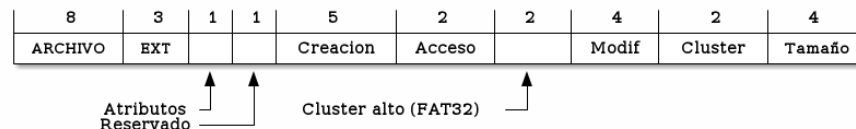
Figura 7.1: Formato de la entrada del directorio bajo FAT (Mohammed, 2007).
