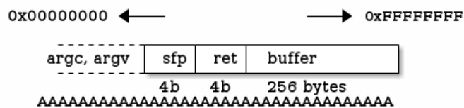
Figura 5.23: Estado de la memoria después del strcpy() .
