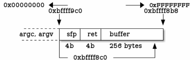
Figura 5.24: Ejecutando el código arbitrario inyectado al buffer.
