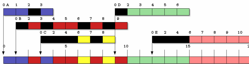
Figura 4.11: Ronda egoísta (SRR) con a = 2 y b = 1 .
