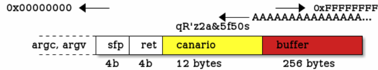
Figura 5.25: Marco de stack con un canario aleatorio protector de 12 bytes (qR' z2a&5f50s): si este es sobrescrito por un buffer desbordado, se detendrá la ejecución del programa.
