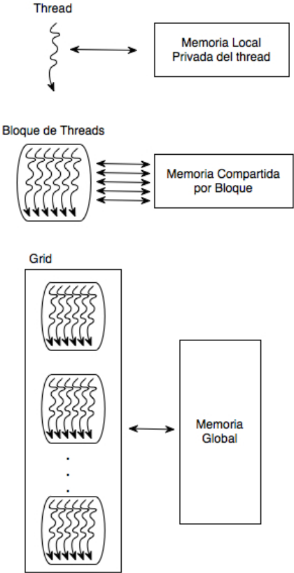
Figura 3.1. Threads y jerarquía de memoria
