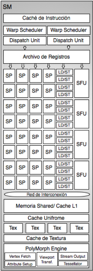
Figura 2.13. Arquitectura de un SM de GF100
