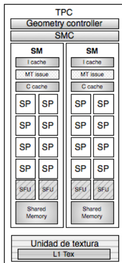
Figura 2.6. Arquitectura de un TPC
