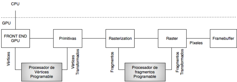
Figura 2.4. Pipeline gráfico programable
