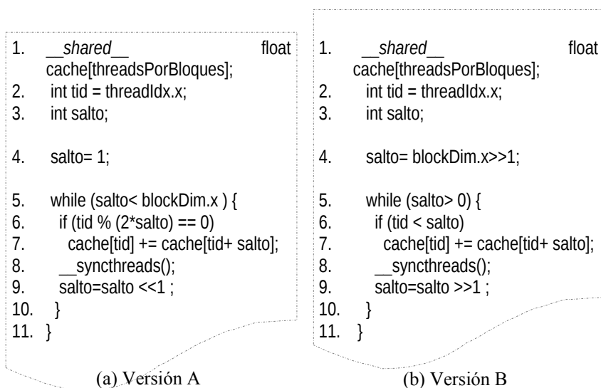
Figura 5.2. Dos versiones de la reduc_sum()
