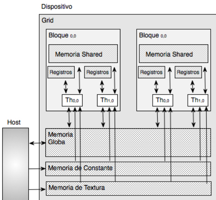
Figura 3.9. Jerarquía de memoria y accesos
