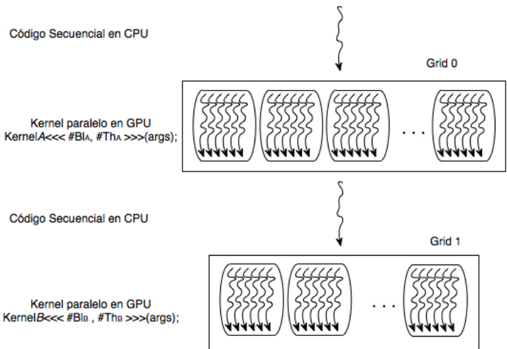
Figura 3.3. Esquema de la estructura de un programa en CUDA
