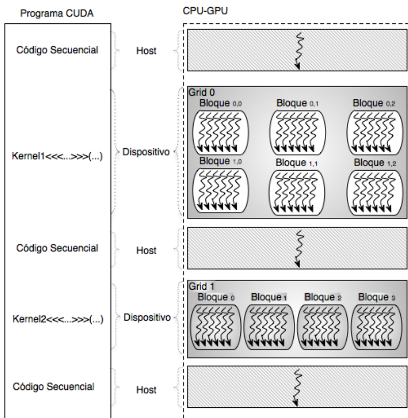
Figura 3.16. Ejecución de un programa CUDA C en un Sistema CPU-GPU
